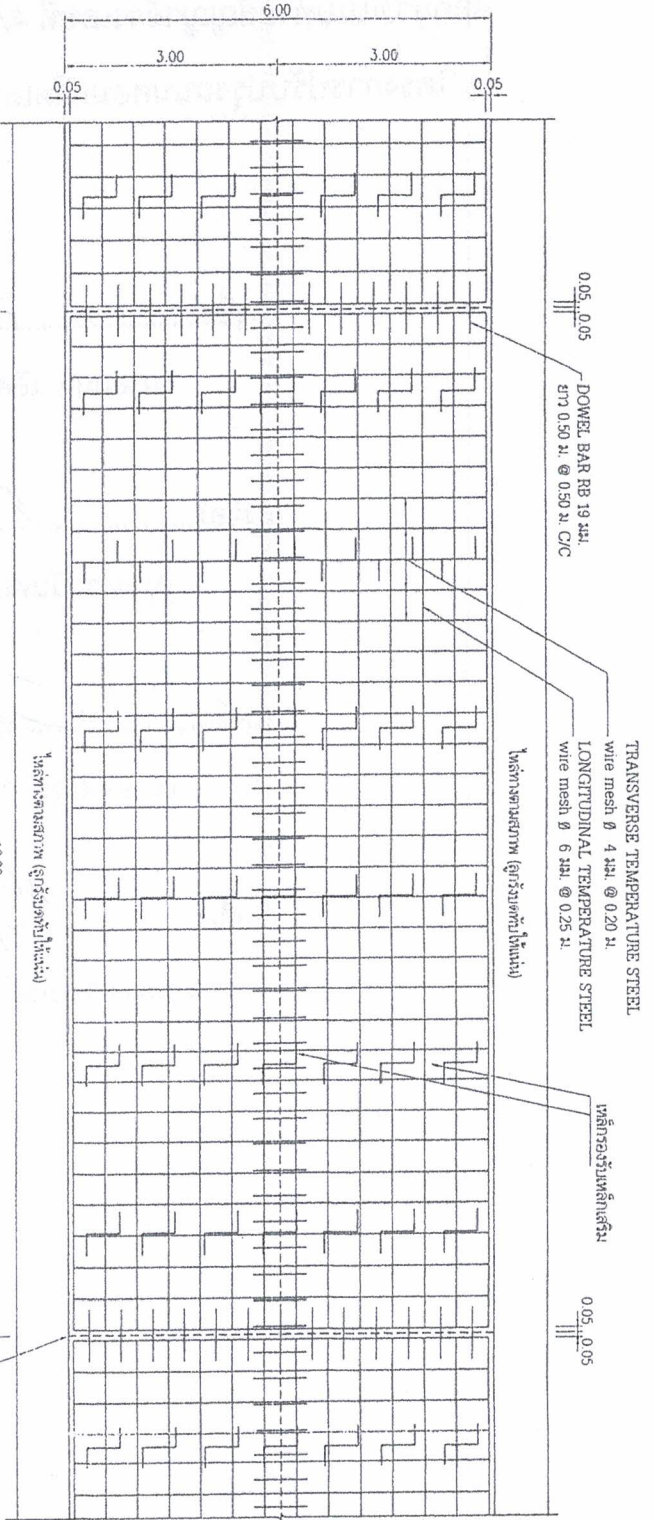
รูปแบบการเสริมกำลังเหล็ก
